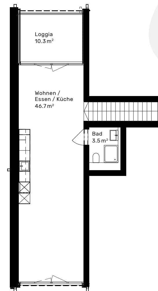
1. Geschoss
