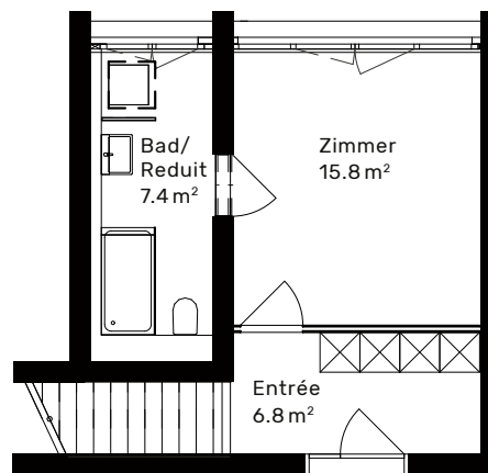
2. Geschoss
