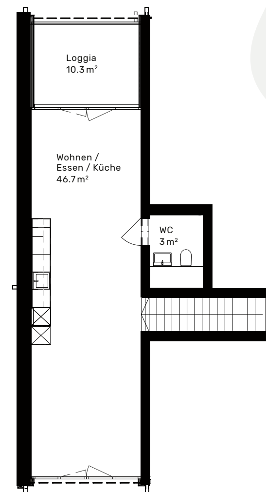
3. Geschoss
