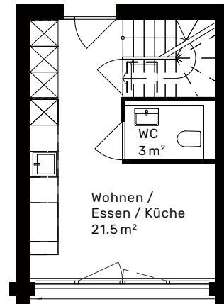
2. Geschoss
