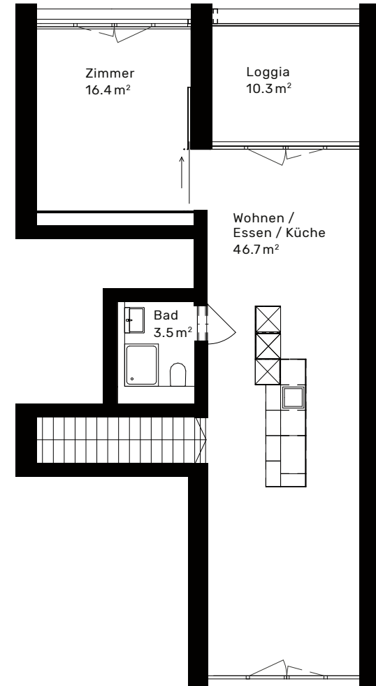
3. Geschoss
