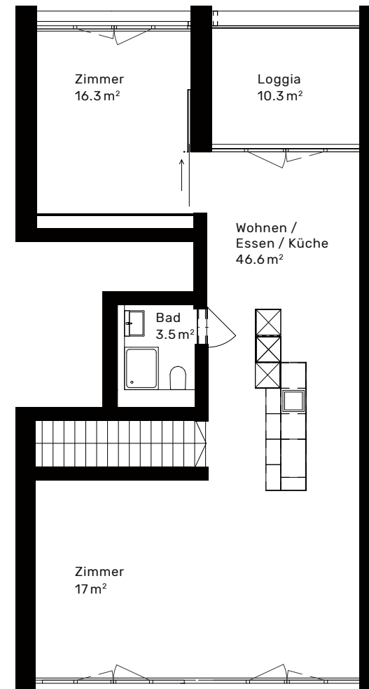
1. Geschoss
